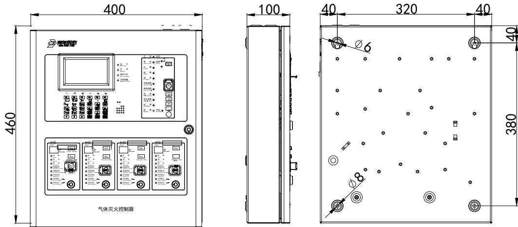
JBF-51S05 尺寸图
