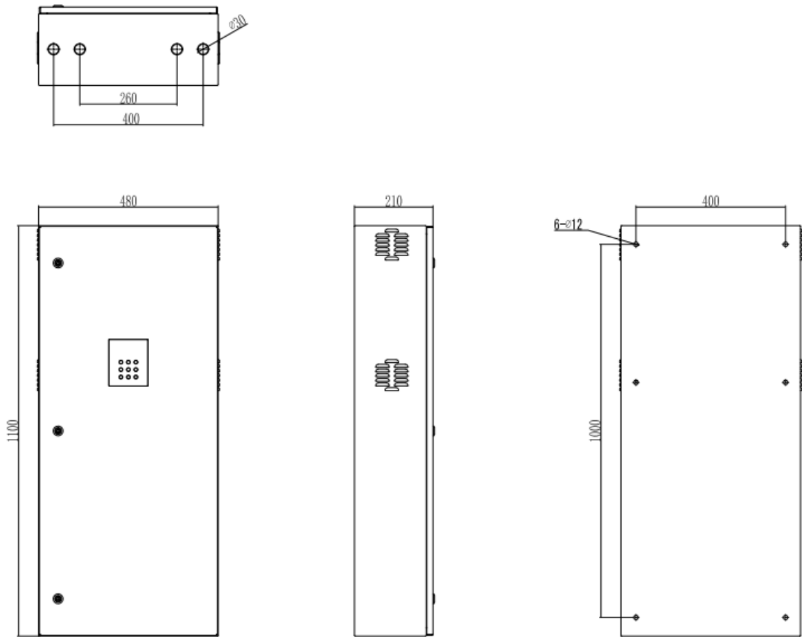
图 2.1 外形尺寸图
