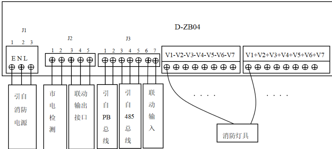
图 3.1 应急照明集中电源接线示意图
