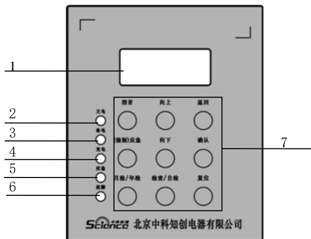
图 4.1 操作面板
