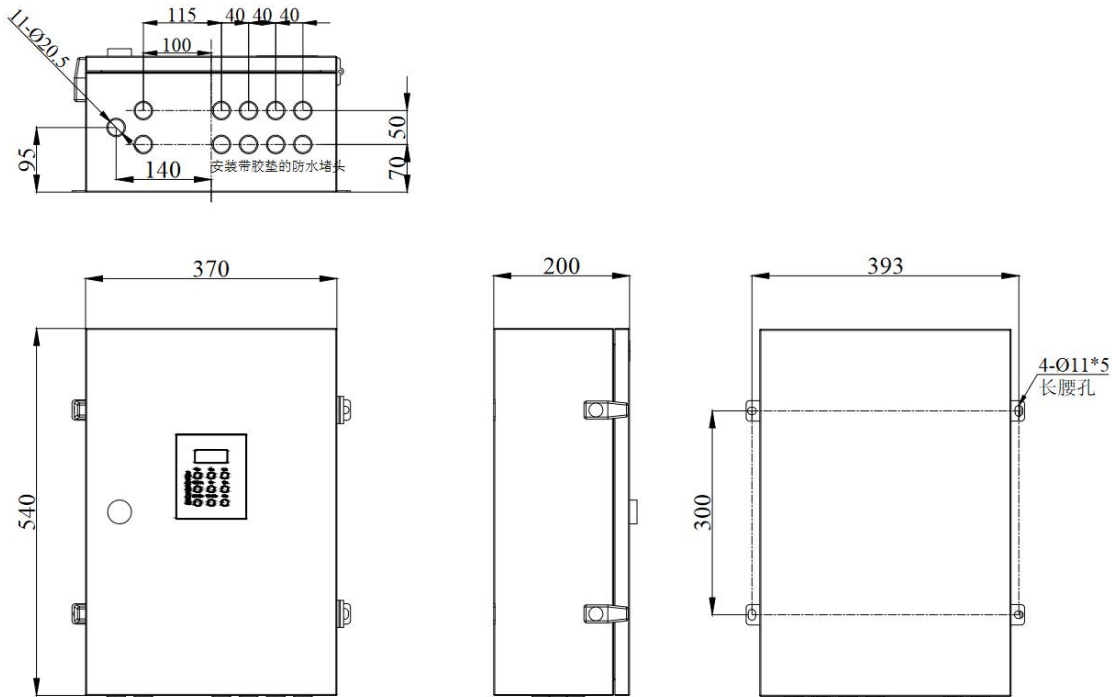
图 2.1 外形尺寸图
