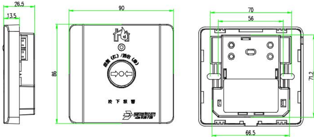
图 4 J-SAP-JBF4125 外形及尺寸图（不含底座）
