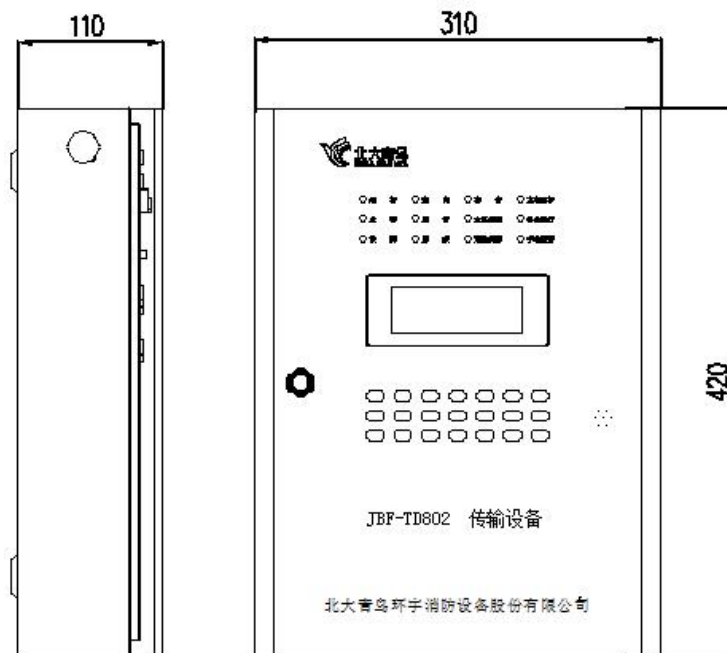
外形尺寸图
