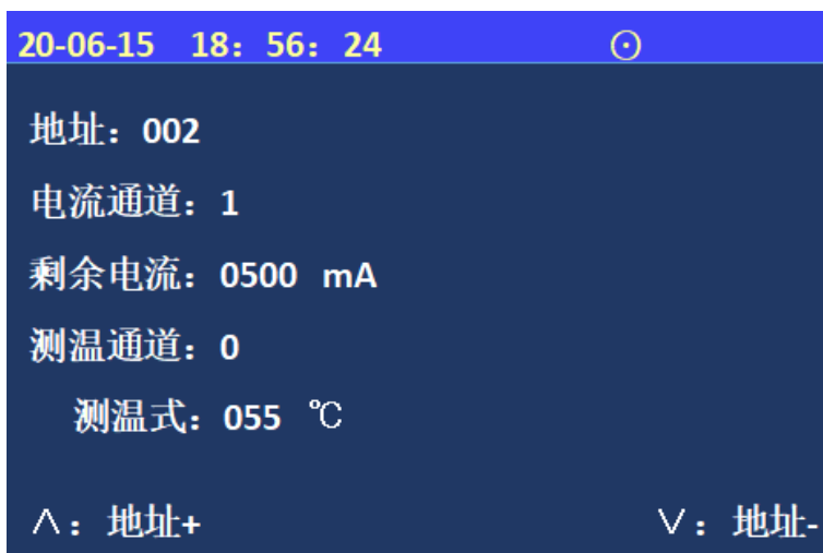
图 5-1-6 查询部件参数
