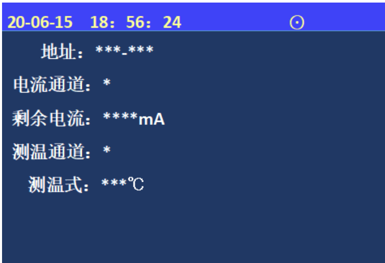
图 5-3-5 设置部件参数
